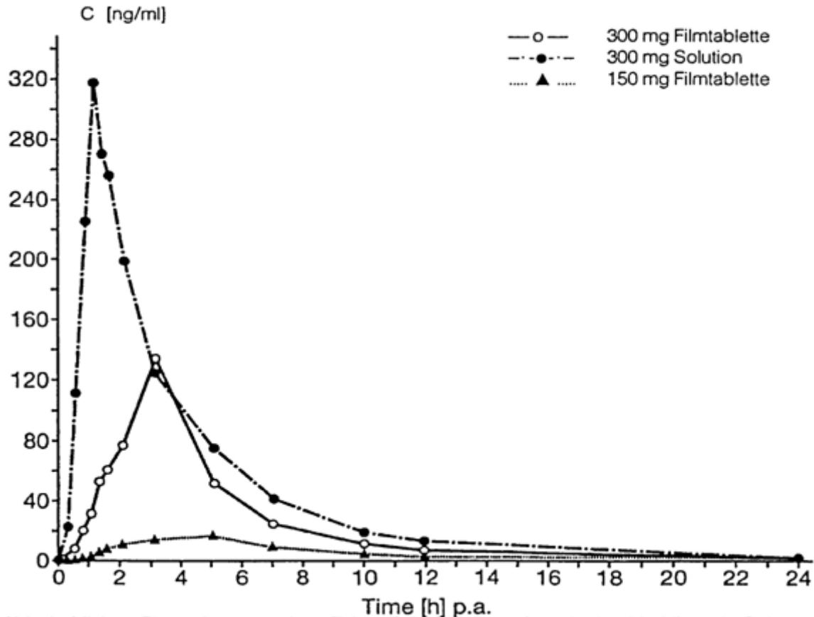
Abb. 1: Mittlere Plasmakonzentrations-Zeitverläufe (als Propafenonhydrochlorid) nach Gabe von 1 Propafenonhydrochlorid 150 mg Filmtablette, 1 Propafenonhydrochlorid 300 mg Filmtablette bzw. 300 mg Propafenonhydrochloridlösung, n = 8.
