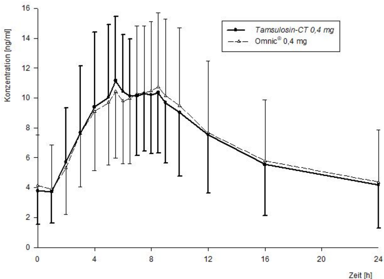
Abb. 1: Arithmetische Mittelwerte und Standardabweichungen der Plasmakonzentration von Tamsulosin nach Gabe von 1 Hartkapsel Tamsulosin-CT 0,4 mg bzw. Referenzpräparat (Omnic® 0,4 mg) im Steady State.
