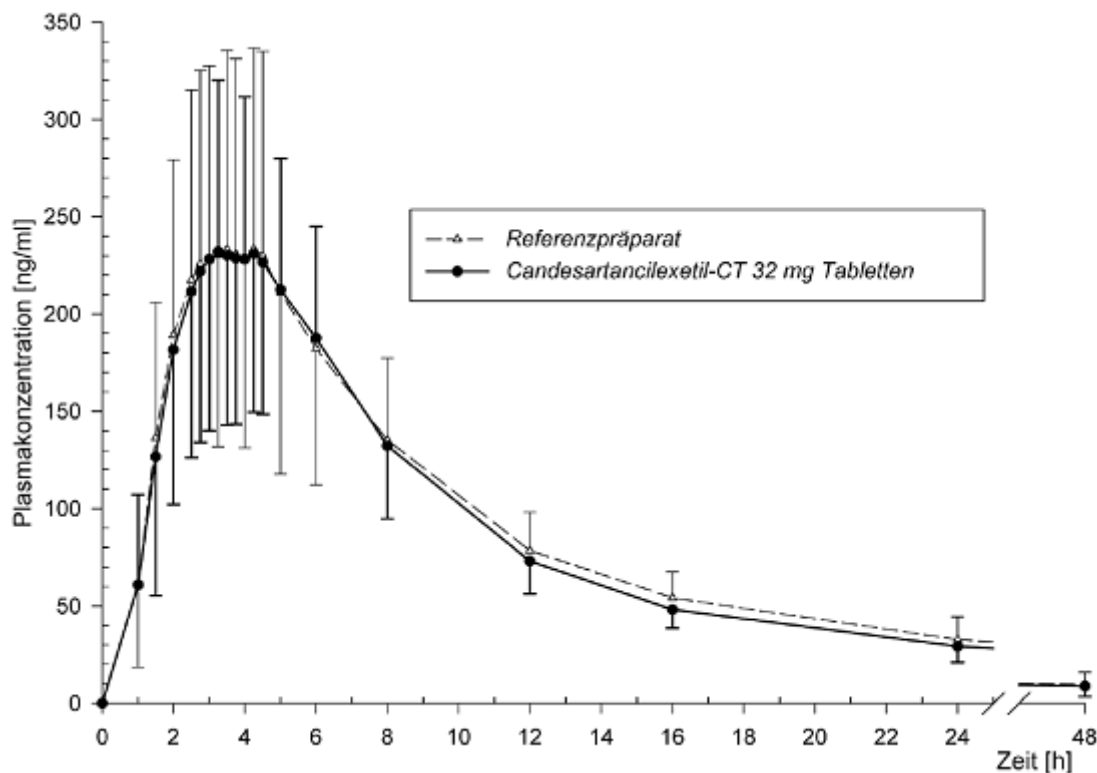
Abb. Mittelwerte und Standardabweichungen der Plasmakonzentration von Candesartan nach Einmalgabe von 1 Tablette Candesartancilexetil-CT 32 mg Tabletten bzw. Referenzpräparat.
