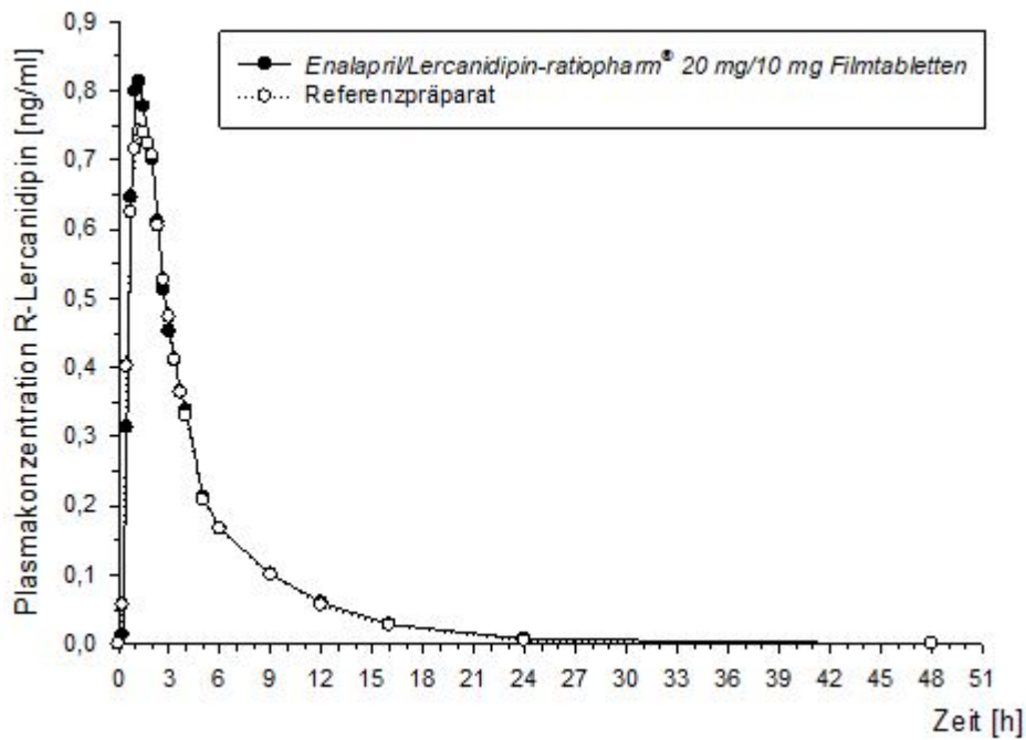
Abb. 3.: Mittelwerte der Plasmakonzentration von R-Lercanidipin nach Einmalgabe von 1 Filmtablette Enalapril/Lercanidipin-ratiopharm ® 20 mg/10 mg Filmtabletten bzw. Referenzpräparat (Zanipress ® ).
