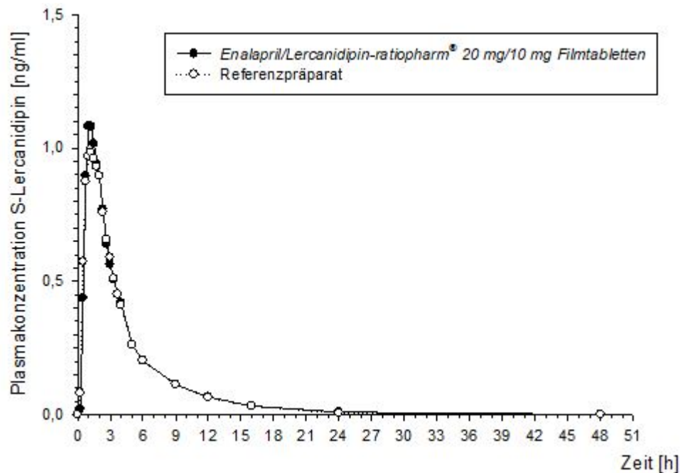
Abb. 2.: Mittelwerte der Plasmakonzentration von S-Lercanidipin nach Einmalgabe von 1 Tablette Enalapril/Lercanidipin-ratiopharm ® 20 mg/10 mg Filmtabletten bzw. Referenzpräparat ( Zanipress ® ).
