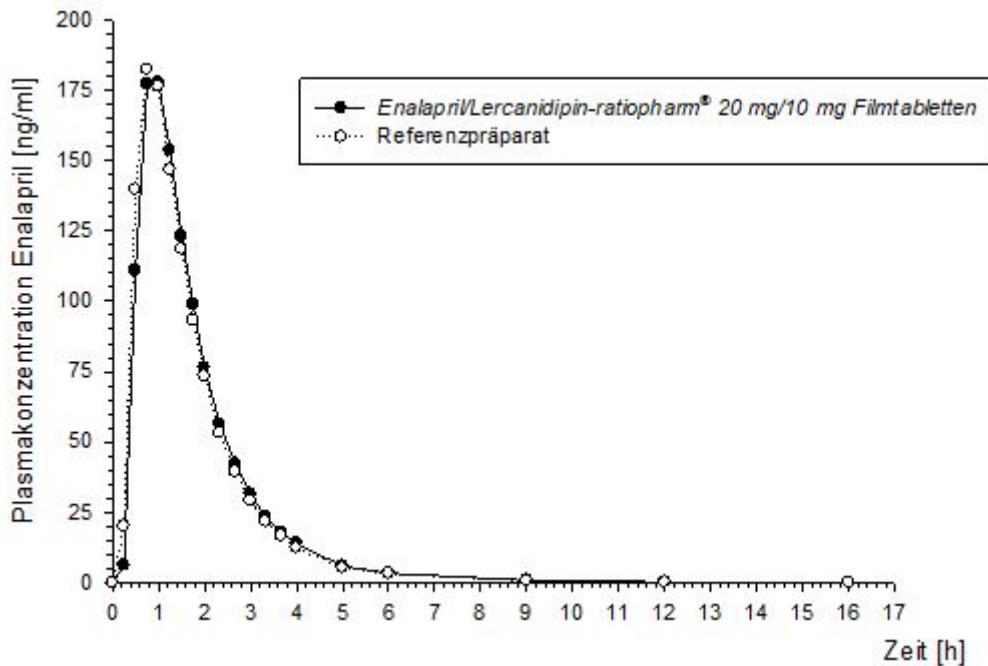
Abb.1: Mittelwerte der Plasmakonzentration von Enalapril nach Einmalgabe von 1 Filmtablette Enalapril/Lercanidipin-ratiopharm® 20 mg/10 mg Filmtabletten bzw. Referenzpräparat (Zanipress®).
