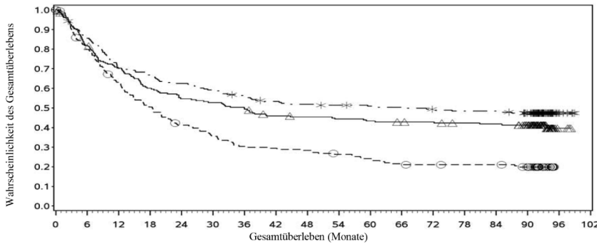
Abbildung 6: Gesamtüberleben nach PD-L1-Expression: 5%-Cut-off (CA209067) – Minimale Nachbeobachtungszeit 90 Monate
