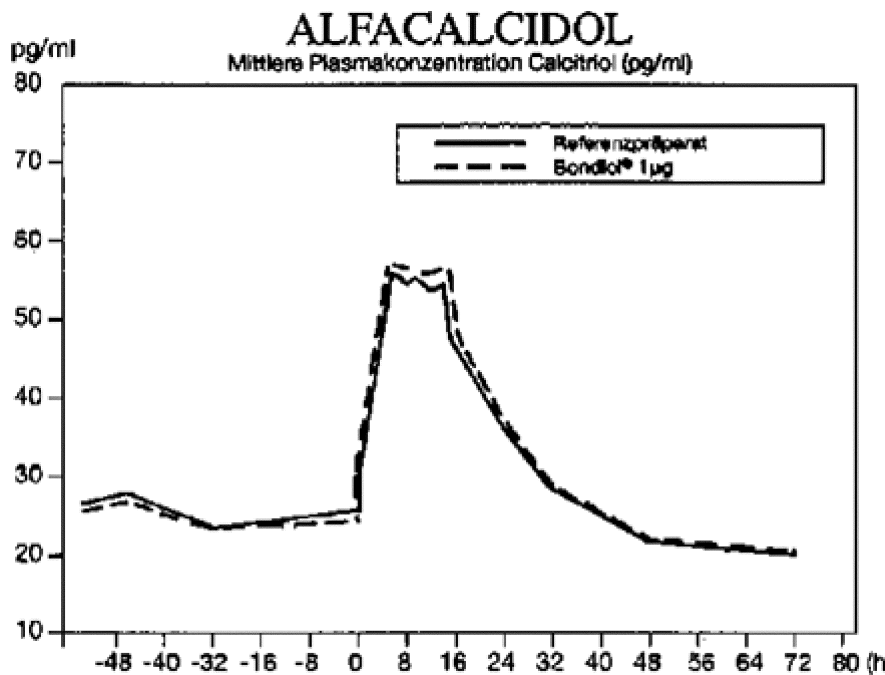
Abbildung 2: Mittlere Plasmaspiegelverläufe von Calcitriol im Vergleich zu einem Referenzpräparat in einem Konzentrations-Zeit-Diagramm (n=16)
