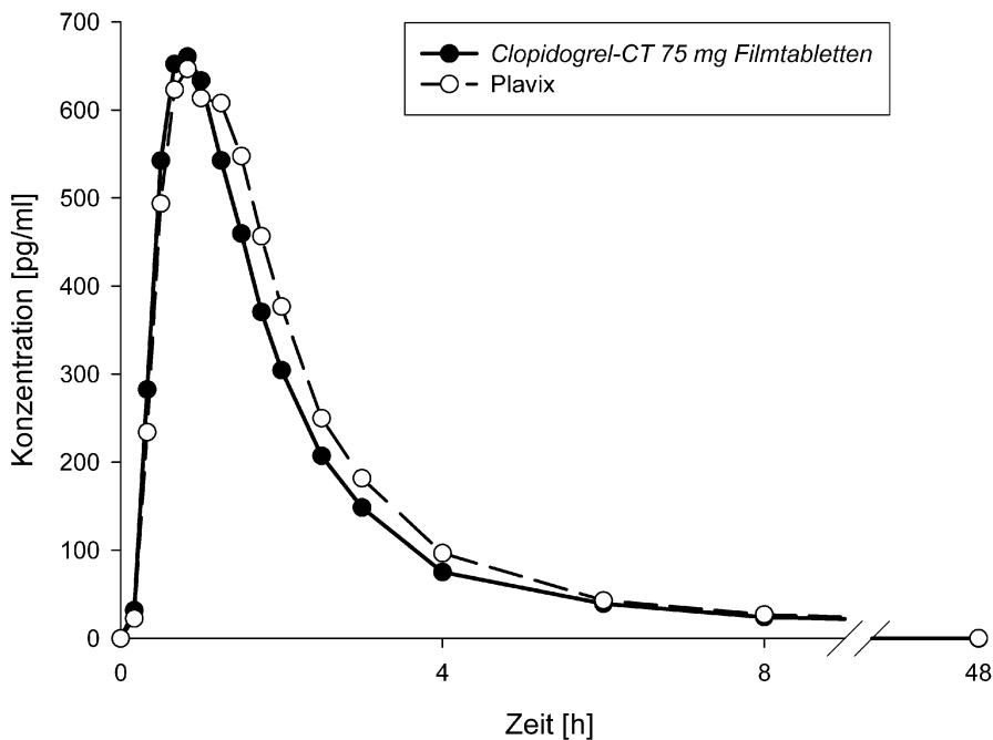
Mittelwerte der Plasmakonzentration von Clopidogrel nach Einmalgabe von 1 Filmtablette Clopidogrel-CT 75 mg Filmtabletten bzw. Plavix®.
